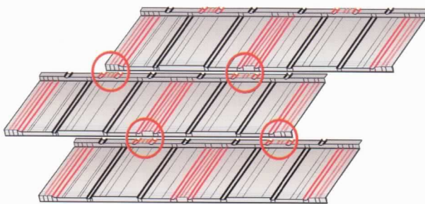
Správný způsob ukládání panelů MetroŠindel
