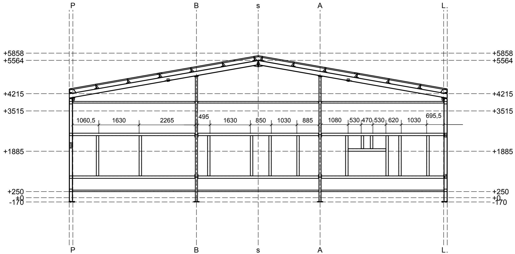
ŠTÍT osa 8 (pohled zvenku)
