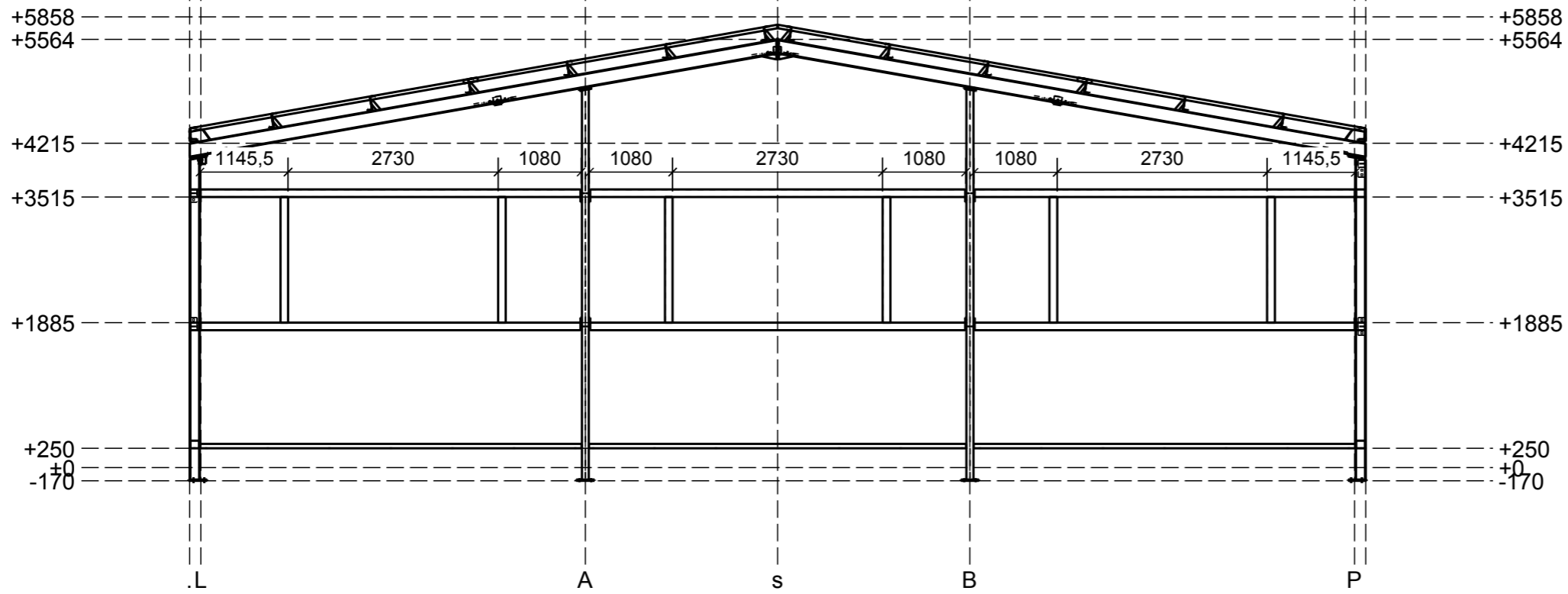
ŠTÍT osa 1 (pohled zvenku)
